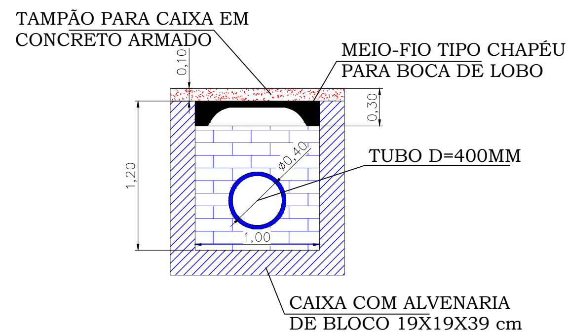
DETALHE DO CORTE "BB" DA DRENAGEM: Esc: ..... 1:30
