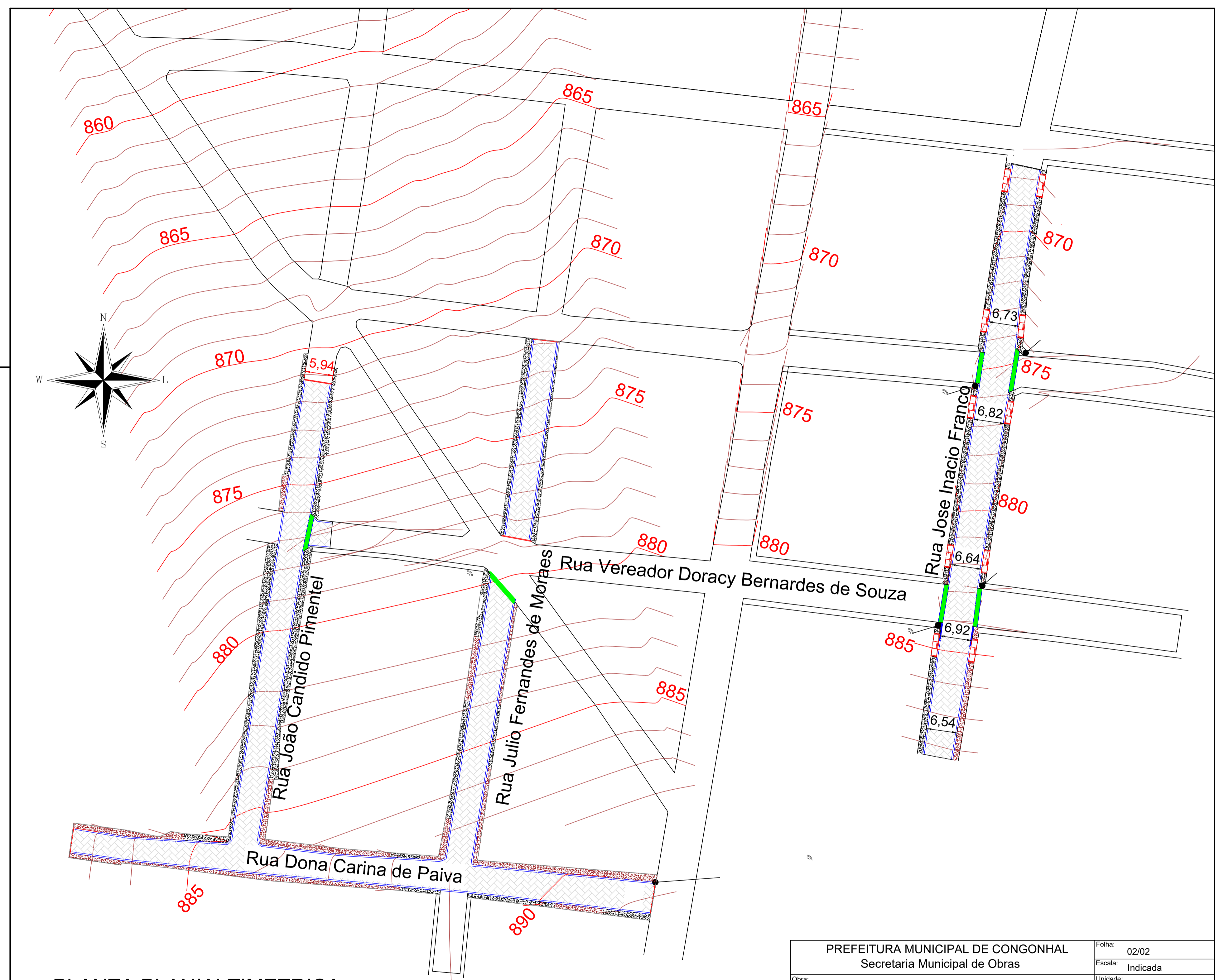
PLANTA PLANIALTIMETRICA Escala: ..... 1:500
